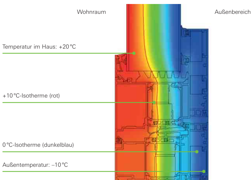
Querschnitt einer hochwärmege­däm­mten Alumi­nium Haustür von Schüco. Der Isothermenverlauf zeigt: Trotz der Minusgrade außen herrscht auch direkt an der Haustür eine angenehme Innentemperatur
