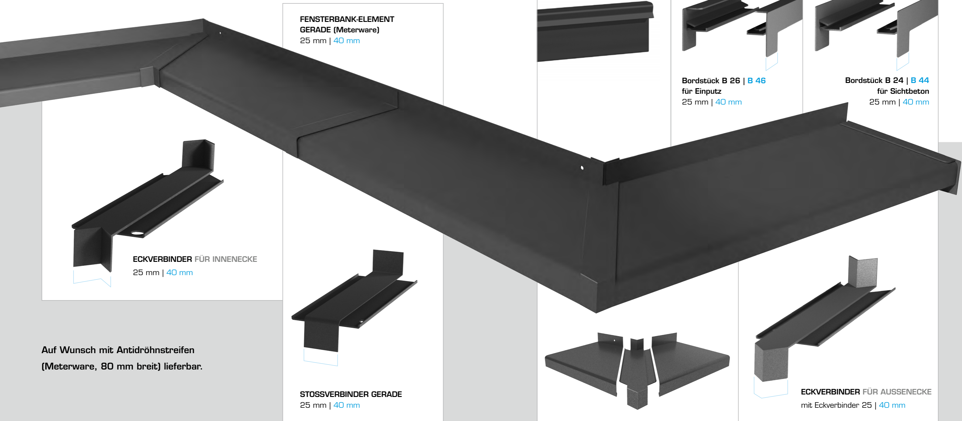
Fensterbankdichtung
